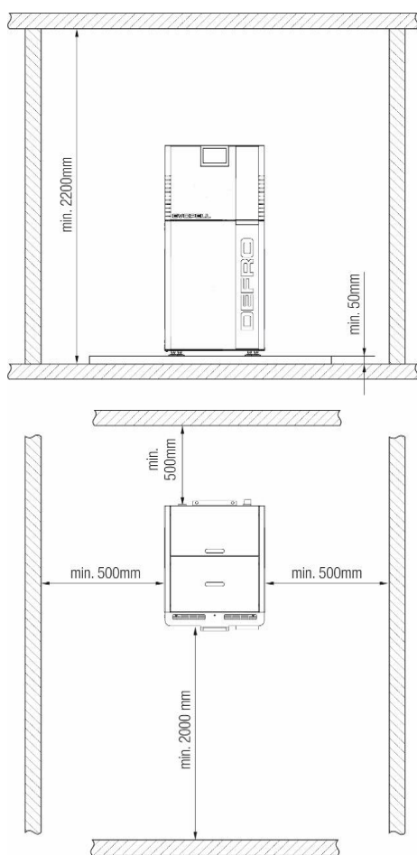
Rysunek 3. Ustawienie kotła w pomieszczeniu kotłowni.
