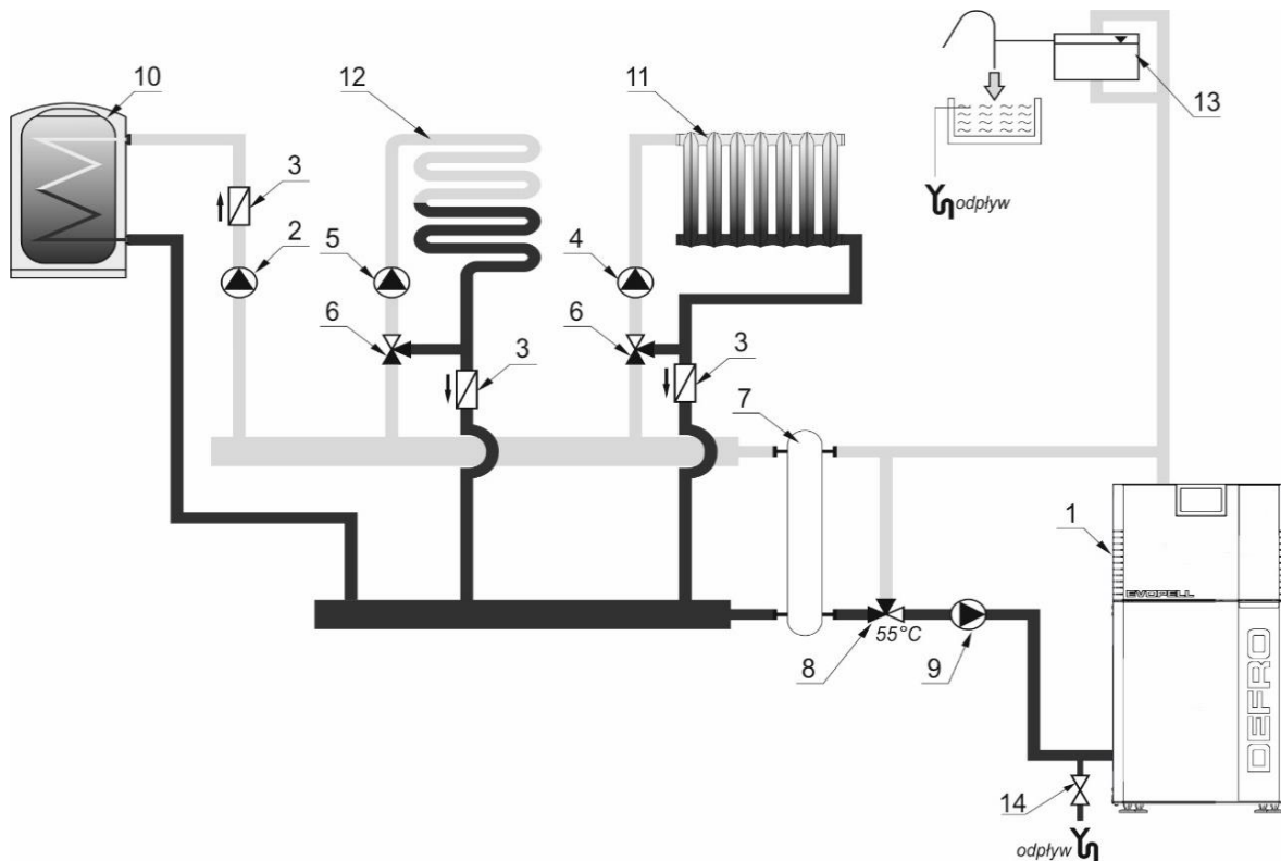
Rysunek 7. Uproszczony schemat instalacji grzewczej systemu otwartego.
