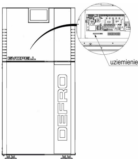
Rysunek 9 Uziemienie kotła.
