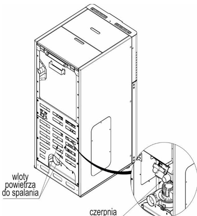
Rysunek 10. Czerpnia powietrza - otwór dolotowy powietrza.
