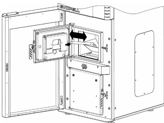
Rysunek 11. Sposób czyszczenia paleniska pelletowego.
