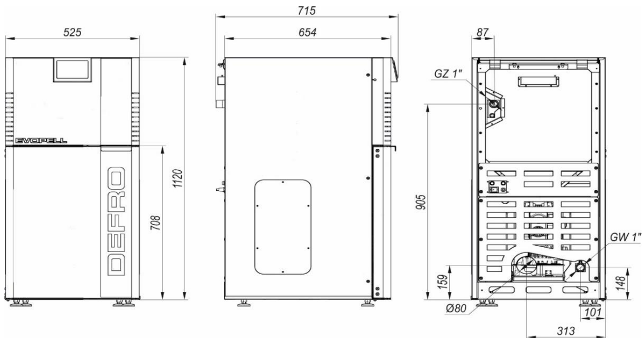
Rysunek 1. Podstawowe wymiary kotła.
