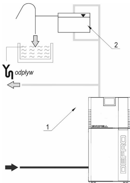
Rysunek 4. Przykładowy schemat zabezpieczeń kotła EVOPELL w układzie otwartym
